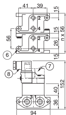
клапан 261
