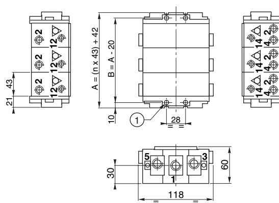
ISO 1 без встроенных регуляторов расхода и встроенных индикаторов давления
