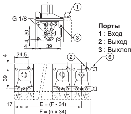
Клапан 263 на соединяемой плите
