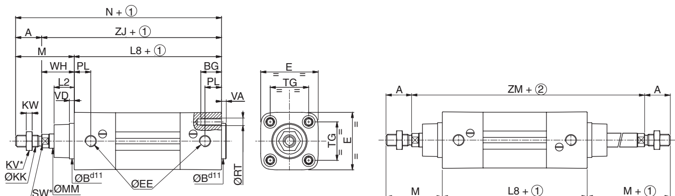
Пневмоцилиндры со стяжными шпильками – серия 450
