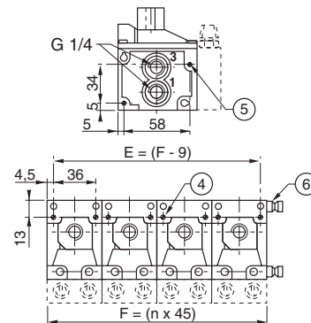
Клапан 264 на соединяемой плите
