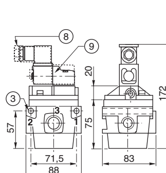
клапан 284
