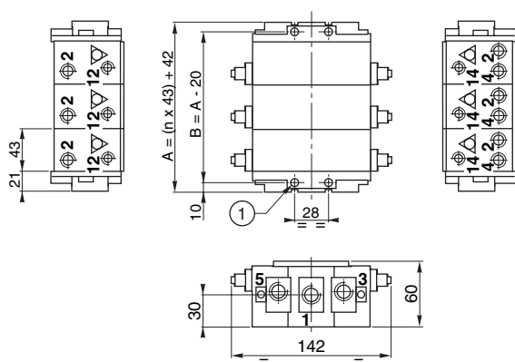
ISO 1 со встроенными регуляторами расхода и встроенными индикаторами давления
