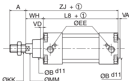
Пневмоцилиндры со стяжными шпильками – серия 450
