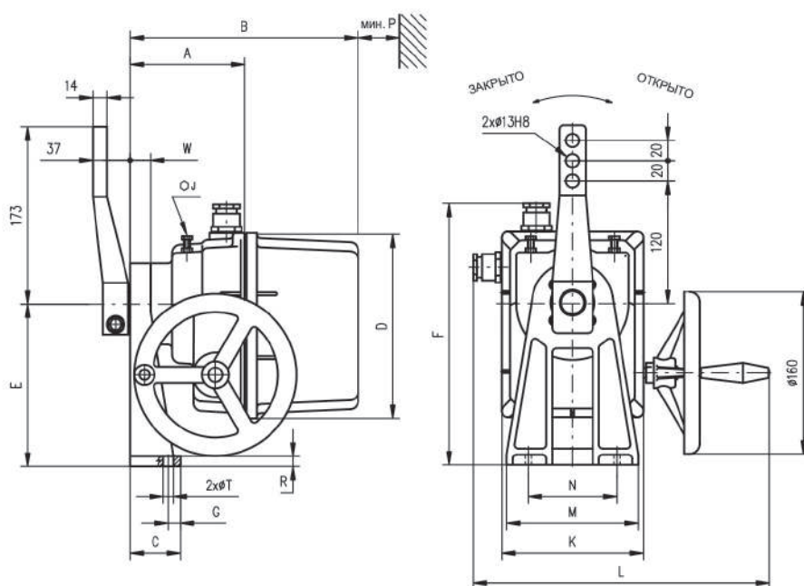
Regada SP 2 — аналог электропривода МЭО 100
