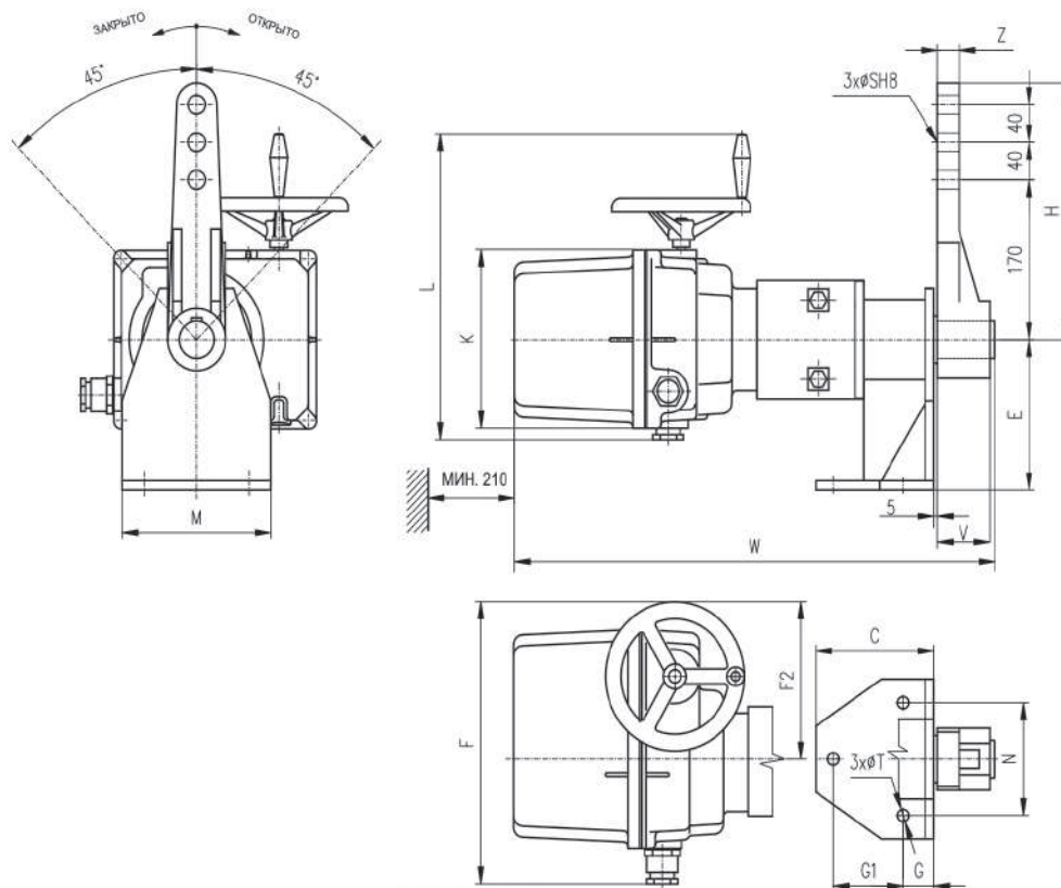
Regada SP 2.3 — аналог электропривода МЭО 250
